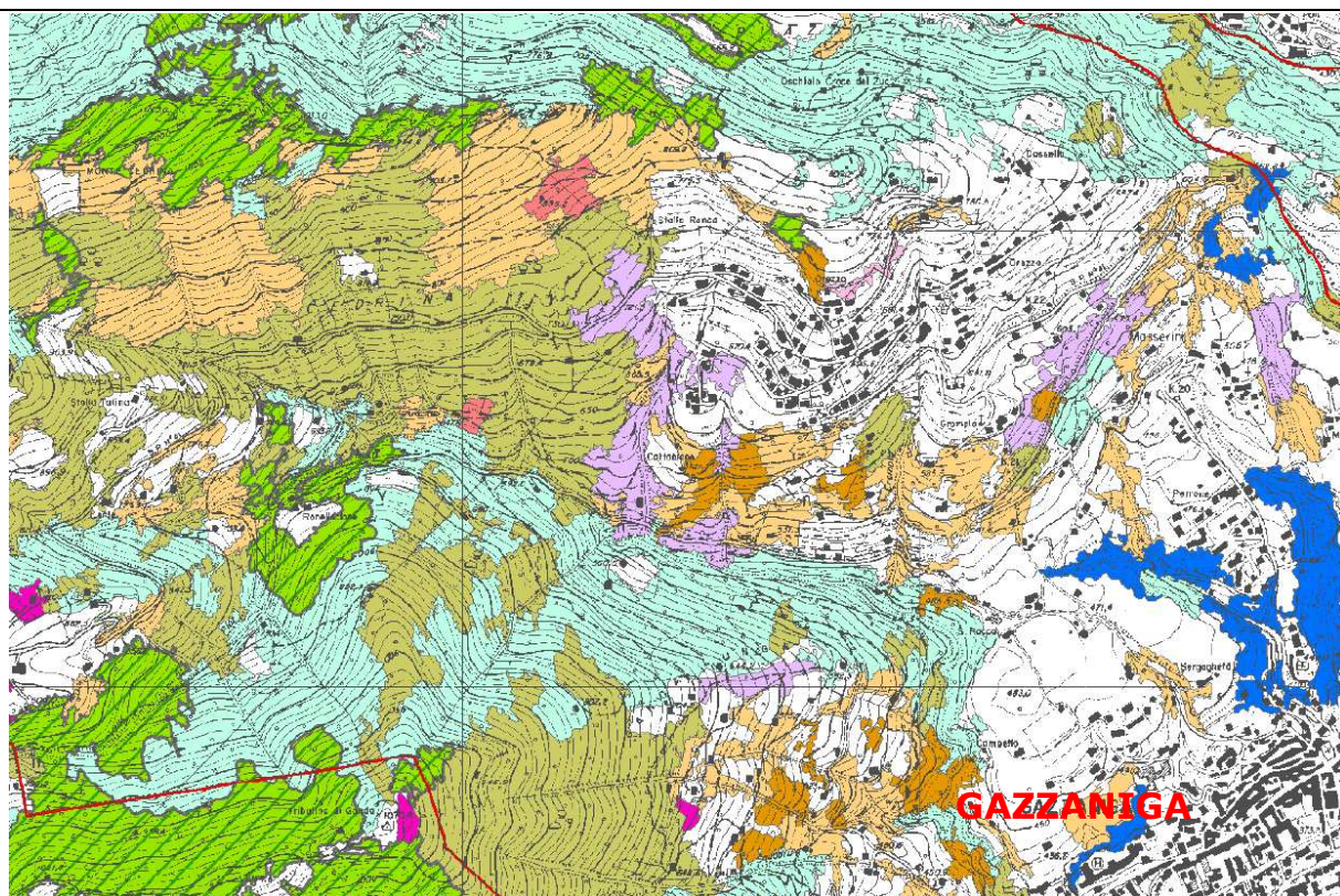
Figura 05 – Il bosco (aree con retino colorato semitrasparente) secondo la “Carta dei Tipi Forestali” del PIF della CM Valle Seriana (settore medio-bassa Valle Seriana). In colore verde marcio è indicata la tipologia forestale del Castagno dei substrati carbonatici dei suoli mesici, in colore marroncino la tipologia dell’Orno-ostrieto tipico, in azzurro chiaro quella dell’Acero-frassinetto tipico, in verde vivo barrato obliquamente quella della Faggeta submontana dei substrati carbonatici, in violetto la tipologia del Betuleto e corileto, in blu vivo il Robinieta misto (immagine non in scala).
